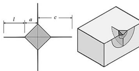
ب- ترک نوع نیم-سکه‌ای الف- اثر سوزن ویکرز و طول ترک
