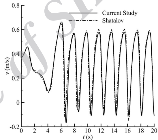
Fig. 6 Comparison of time variation of the v -velocity at x = 2.0 , y = 0.0 behind the NACA0012, \alpha = 20^\circ and Re = 800 [7] شکل 6 مقایسه تغییرات سرعت عمودی v در موقعیت x = 2.0 , y = 0.0 پشت هیدروفویل NACA0012 بر حسب زمان، \alpha = 20^\circ و Re = 800 [7]
