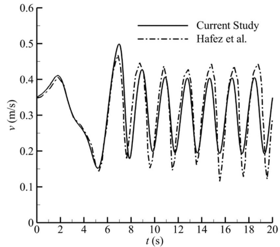
Fig. 5 Comparison of time variation of the v -velocity at x = 3.0 , y = 0.0 behind the NACA0012, \alpha = 20^\circ and Re = 800 [28] شکل 5 مقایسه تغییرات سرعت عمودی v در موقعیت x = 3.0 , y = 0.0 پشت هیدروفویل NACA0012 بر حسب زمان، \alpha = 20^\circ و Re = 800 [28]
