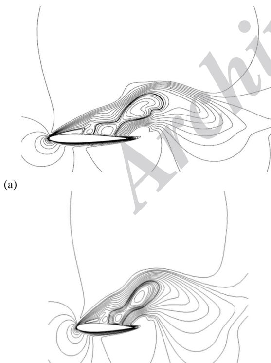
Fig. 8 u -velocity contours on the NACA0012, \alpha = 20^\circ , Re = 800 and time = 5 (a): Hafez et al [28] (b): Current study شکل 8 خطوط همتراز سرعت افقی u هیدروفویل NACA0012، \alpha = 20^\circ ، Re = 800 و زمان t = 5 : (a) حافظ [28]؛ (b) مطالعه‌ی حاضر
