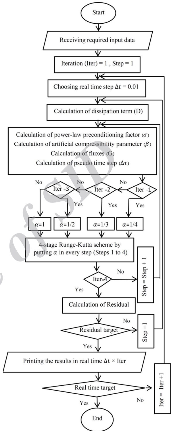
Fig. 1 The flowchart of the computational algorithm شکل 1 روندنمای الگوریتم محاسباتی
