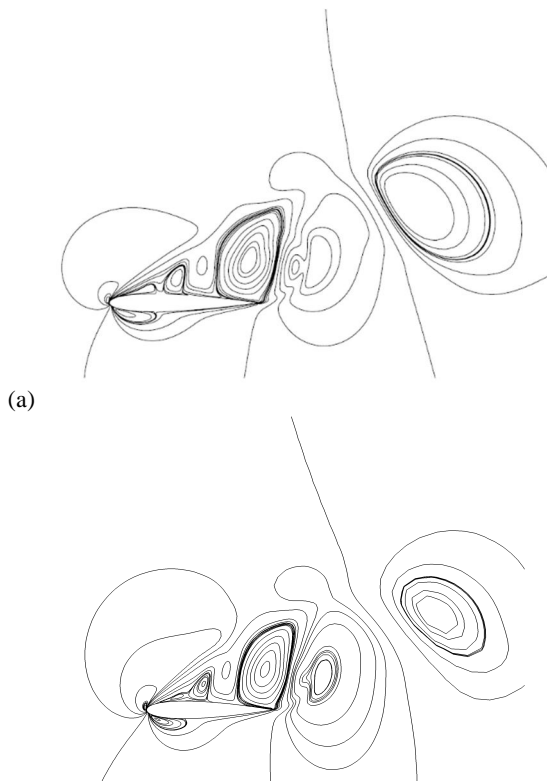
Fig. 7 v -velocity contours on the NACA0012, \alpha = 20^\circ , Re = 800 and t = 5 (a): Hafez et al [28] (b): Current study شکل 7 خطوط همتراز سرعت عمودی v هیدروفویل NACA0012، \alpha = 20^\circ ، Re = 800 و زمان t = 5 : (a) حافظ [28]؛ (b) مطالعه‌ی حاضر
