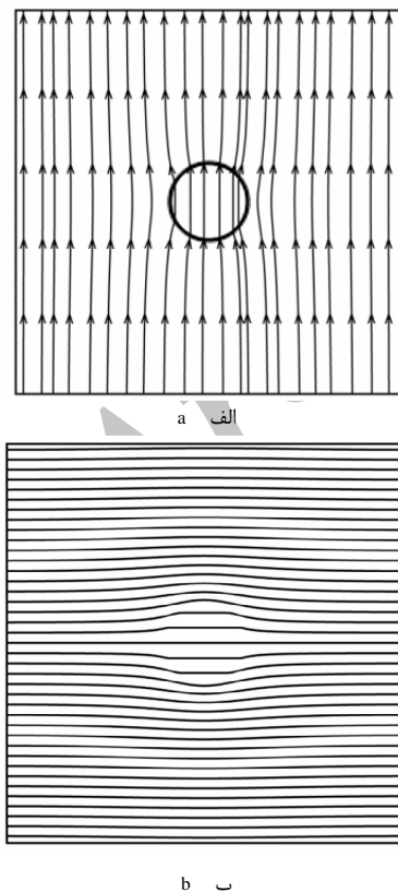
Fig. 6 a: The magnetic field lines b: magnetic potential for permeable circle placed in a uniform magnetic field in y direction شکل 6 نمودار(الف): خطوط میدان مغناطیسی ب: پتانسیل مغناطیسی) برای دایره نفوذپذیر تحت میدان مغناطیسی یکنواخت در جهت عمود
