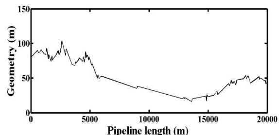
Fig. 1 First 20 kilometers of Golkhari to Binak pipeline profile شکل 1 20 کیلومتر اول از پروفایل خط لوله گلخاری به بینک
