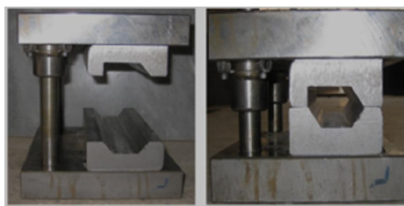
Fig. 5 The two-piece liquid impact forming die شکل 5 قالب شکل‌دهی با ضربه مایع متشکل از دو قطعه
