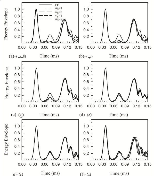
Fig. 9 Envelope energy relative to the field nodes: a) 100 b) 200 c) 300 d) 400 e) 500 f) 1000 for \alpha_s = \{1, 2, 4, 8\} ( \alpha_c = 1, n_g = 3000, m = 3 ) شکل 9 پوش انرژی نسبت به تعداد نقاط میدانی الف) 100 ب) 200 ج) 300 د) 400 ه) 500 و) 1000 به ازاء \alpha_s = \{1, 2, 4, 8\} ( \alpha_c = 1, n_g = 3000, m = 3 )
