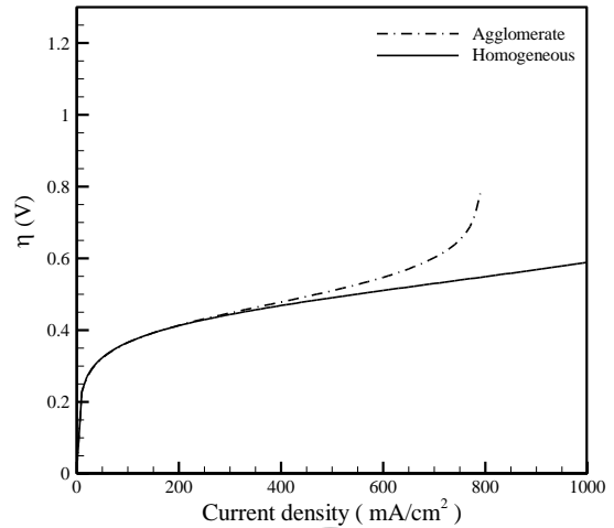
Fig 8 Comparison activation loss homogeneous & agglomerate model شکل 8 مقایسه افت فعال‌سازی مدل هموزن و توده‌ای
