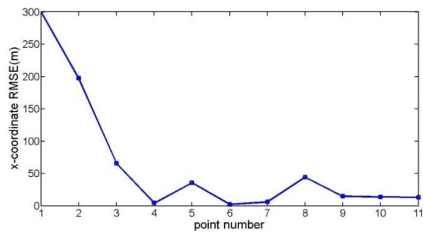
Fig. 12 X-coordinate RMSE of estimated target points شکل 12 مقدار RMSE مختصات x تخمین زده شده نقاط هدف
