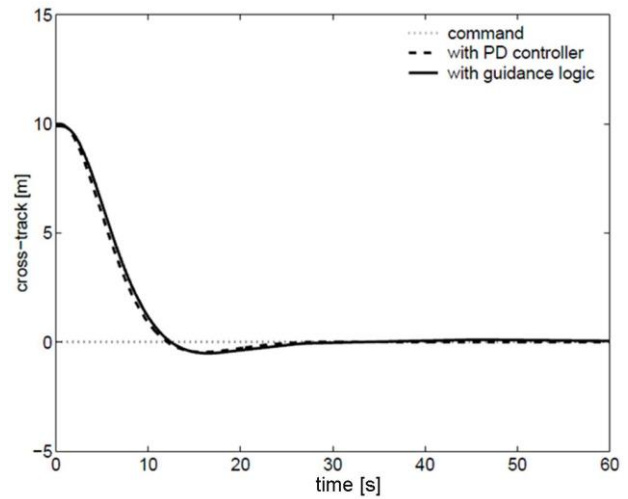
Fig. 10 Tracking straight path شکل 10 تعقیب مسیر مستقیم
