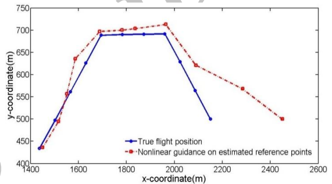
Fig. 11 Tracking desired path with recommended nonlinear guidance on estimated reference points شکل 11 تعقیب مسیر مورد انتظار توسط هدایت غیرخطی پیشنهادی در نقاط مرجع تخمین زده شده
