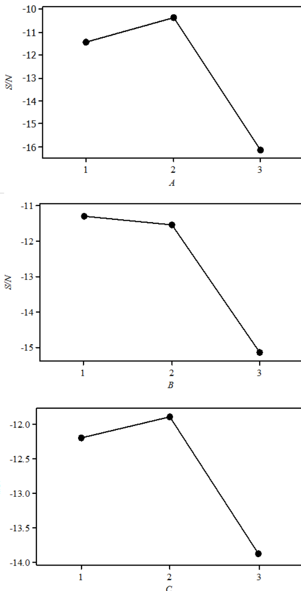
شکل 5 نمودار نسبت سیگنال به نویز برای درصد تخلخل
