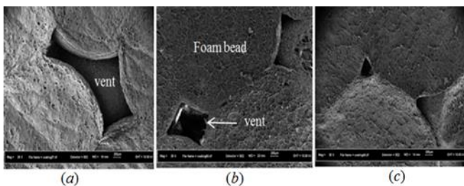
شکل 6 منافذ بین دانه‌های فوم
