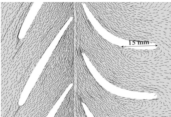
B. Optimized geometry ب هندسه بهبود یافته
