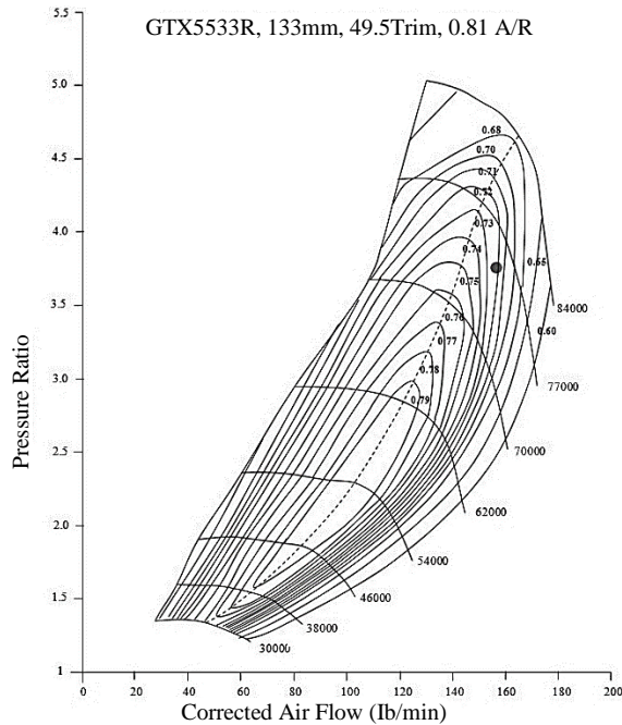
Fig. 9 The well-chosen LP turbocharger compressor map [9] شکل 9 نقشه عملکردی کمپرسور فشار پایین معرفی شده توسط نرم‌افزار [9]
