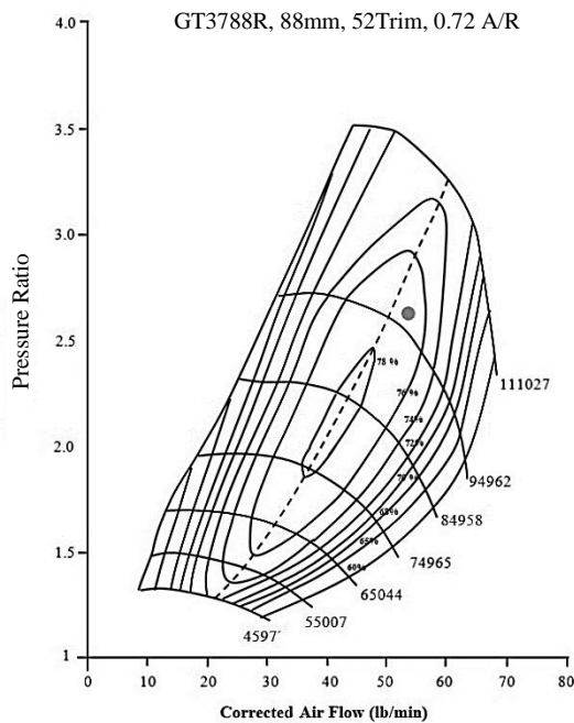
Fig. 10 The well-chosen IP turbocharger compressor map [9] شکل 10 نقشه عملکردی کمپرسور فشار متوسط معرفی شده توسط نرم‌افزار [9]
