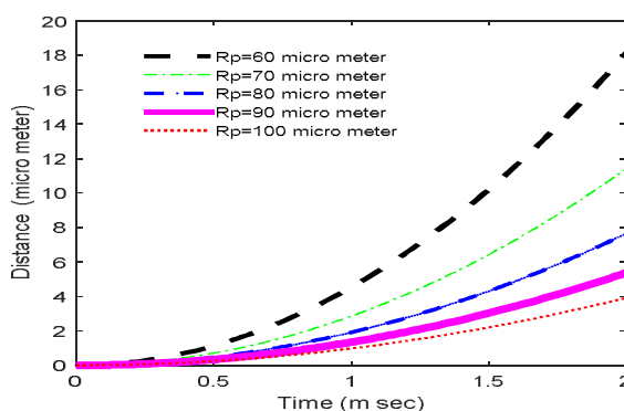
نمودار ۱) جابه‌جایی ذرات در مدت زمان ۲ میلی‌ثانیه در مدل اصطکاکی کولمب
