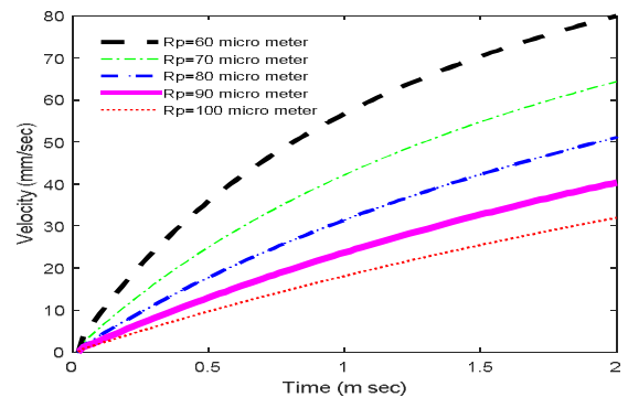
نمودار ۶) سرعت ذرات در مدت زمان ۲ میلی‌ثانیه در مدل اصطکاکی لاگره
