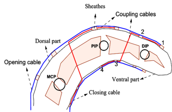
شکل ۶ طرح چیدمان سیستم کابلی جدید کابلی پیشنهاد شده در این مقاله
