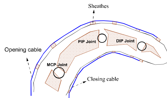
شکل ۱) طرح چیدمان سیستم کابلی انگشتان رباتیک موجود
