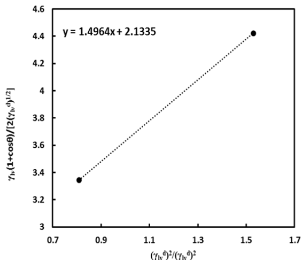
نمودار ۶) محاسبه انرژی سطحی به روش میانگین هندسی برای سطح کلسیت پیرشده در نانوسیال ۵
