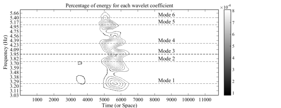
Fig. 12 The time-frequency presentation obtained from the radial output records at the crest level during 2008 earthquake شکل 12 نمایش زمان-فرکانس به دست آمده از رکوردهای شعاعی خروجی در تراز تاج طی زلزله 2008
