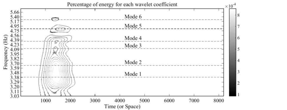
Fig. 10 The time-frequency presentation obtained from the radial output records at 80% height of the dam during 2001 earthquake شکل 10 نمایش زمان-فرکانس به دست آمده از رکوردهای شعاعی خروجی در تراز 80% ارتفاع سد طی زلزله 2001
