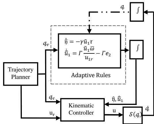
Fig. 3 System control diagram with adaptive slips estimator شکل 3 دیاگرام کنترلی سیستم به همراه تخمینگر تطبیقی لغزش ها
