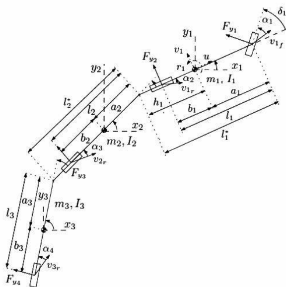
Fig. 9 Simple model of long articulated vehicle شکل 9 مدل ساده از خودروی طولی مفصلی
