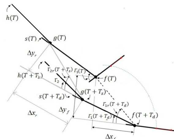
Fig. 8 Desired articulation angles for articulated long vehicle شکل 8 زاویه‌های مفصل مرجع برای خودروی طولی مفصلی
