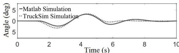
Fig. 6 Comparison of first articulation angle in Matlab and Trucksim شکل 6 مقایسه زاویه مفصل اول در نرم افزار متلب و تراکسیم
