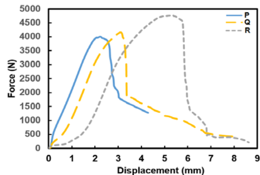
نمودار ۶) منحنی نیرو- جابجایی نمونه‌های جوشکاری‌شده در سرعت دوران ۲۰۰۰rpm و زمان‌های دوران مختلف
