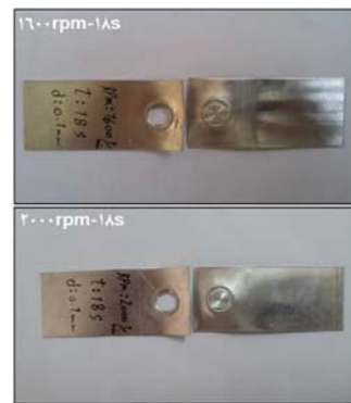
شکل ۱۰) تصویر ماکروسکوپی از نمونه‌های جوشکاری شده در زمان دوران ۱۸S و سرعت‌های دوران ۱۶۰۰rpm و ۲۰۰۰rpm
