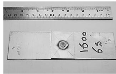
شکل ۴) نمونه آماده‌سازی شده برای آزمون کشش برش
