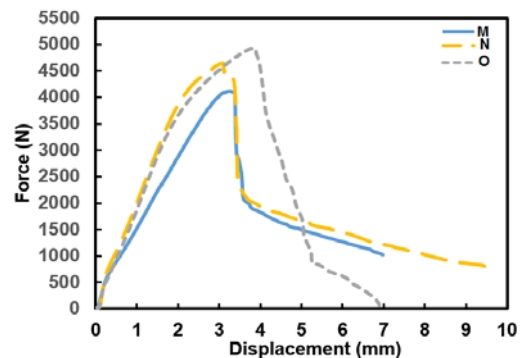
نمودار ۵) منحنی نیرو- جابجایی نمونه‌های جوشکاری‌شده در سرعت دوران ۱۶۰۰rpm و زمان‌های دوران مختلف
