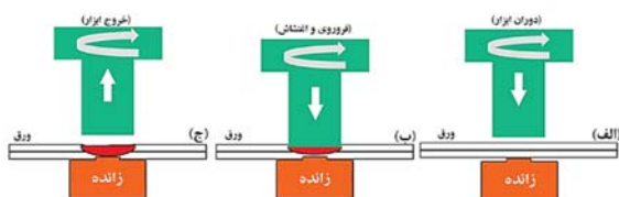
شکل ۳ تصویر شماتیک از مراحل فرآیند PFSSW شامل: (الف) دوران، (ب) فروروی و اغتشاش (ج) خارج شدن ابزار
