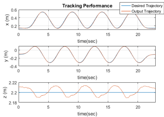
نمودار (۱) کارایی ربات در ردیابی مسیر مطلوب.
