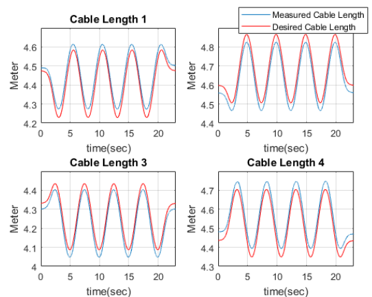
نمودار (۳) مقایسه تغییرات طول کابل مطلوب با تغییرات طول کابل اندازه‌گیری شده
