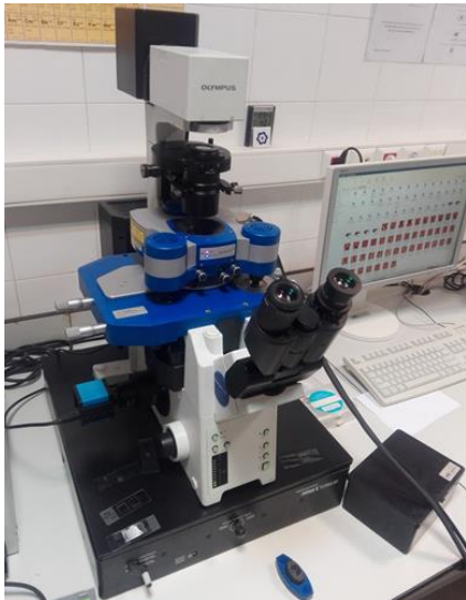
شکل ۷) میکروسکوپ نیروی اتمی 2 JPK Instruments-NanoWizard برای آزمودن تیرک در محیط آب
