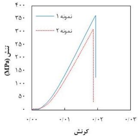
شکل 4 نمودار تنش- کرنش تست کشش نمونه‌های GFRP
