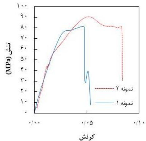
شکل 5 نمودار تنش- کرنش برشی نمونه‌های GFRP
