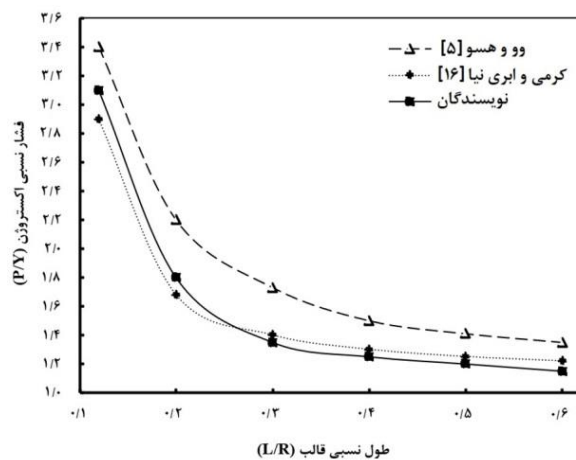
شکل ۱۱ مقایسه فشار فرآیند اکستروژن مقطع شش ضلعی حاصل از روش نویسندگان با پژوهش‌های پیشین
