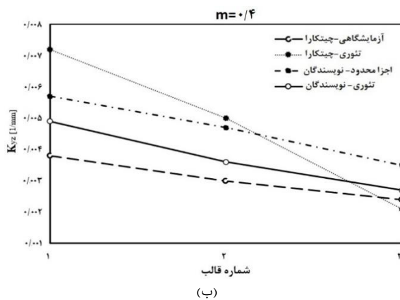
شکل ۱۶) مقایسه انحنای محصول خروجی از قالبها در صفحه yz حاصل از روش نظری و اجزا محدود نویسندگان با نتایج آزمایشگاهی و نظری کلیک و چیتکارا [4] در الف) m=0.2 و ب) m=0.4
