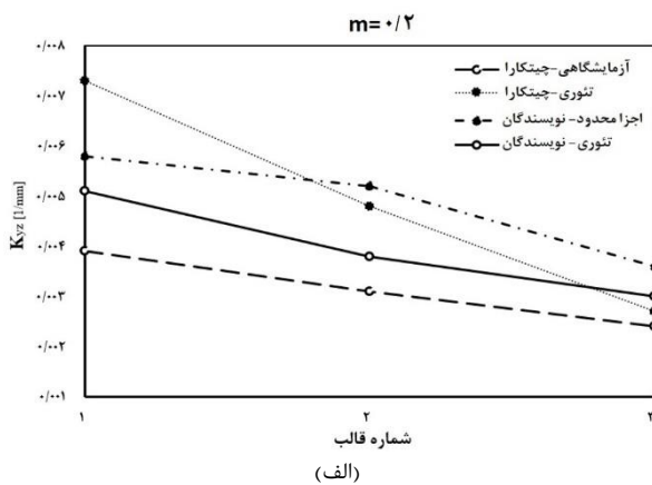
شکل ۱۵) مقایسه انحنای محصول خروجی در صفحه yz در قالبهای شماره ۱ و ۲ و ۳ در الف) m=0.2 و ب) m=0.4
