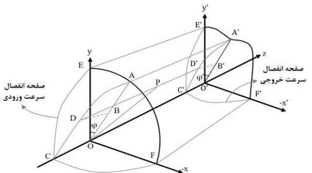
شکل ۳) یک چهارم میدان تغییر شکل برای اکسترودین مقطع دایره به مقطع دلخواه
