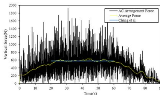
نمودار (۵) اعتبارسنجی نیرو عمودی وارد بر ابزار و مقایسه نتایج عددی و تئوری
