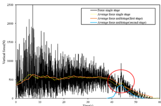
نمودار ۱۳) تأثیر استراتژی بر نیروی متوسط عمودی وارد بر ابزار
