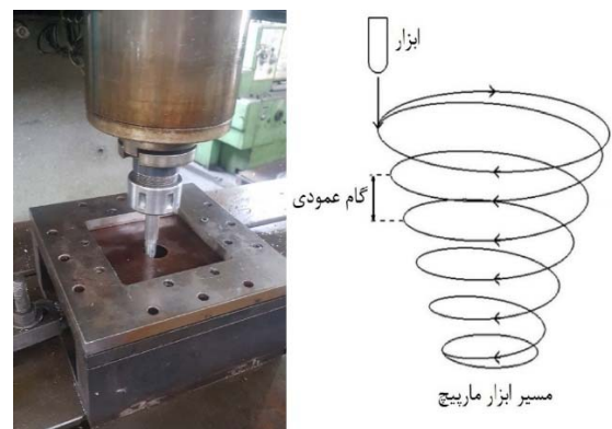
شکل ۲) تجهیزات فرم‌دهی ورق سوراخ‌دار و شماتیک مسیر ابزار
