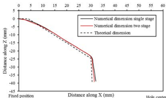
نمودار ۱۱) تأثیر استراتژی بر دقت ابعادی ورق دولایه
