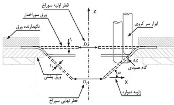
شکل ۳ شماتیک پارامترها و قرارگیری ورق و تجهیزات
