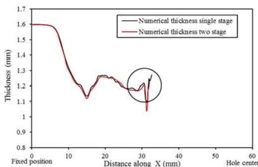
نمودار ۱۲) تأثیر استراتژی بر توزیع ضخامت ورق دولایه
