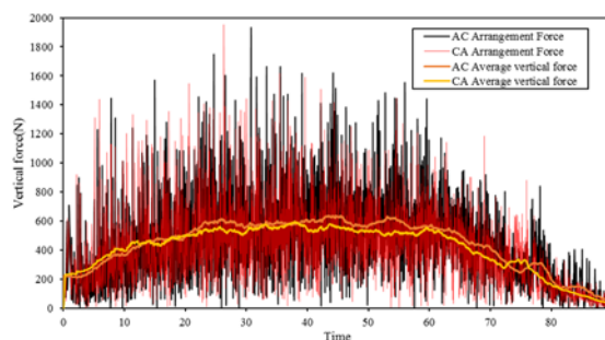
نمودار ۱۰) تأثیر چینش لایه‌ها بر نیروی عمودی وارد بر ابزار
