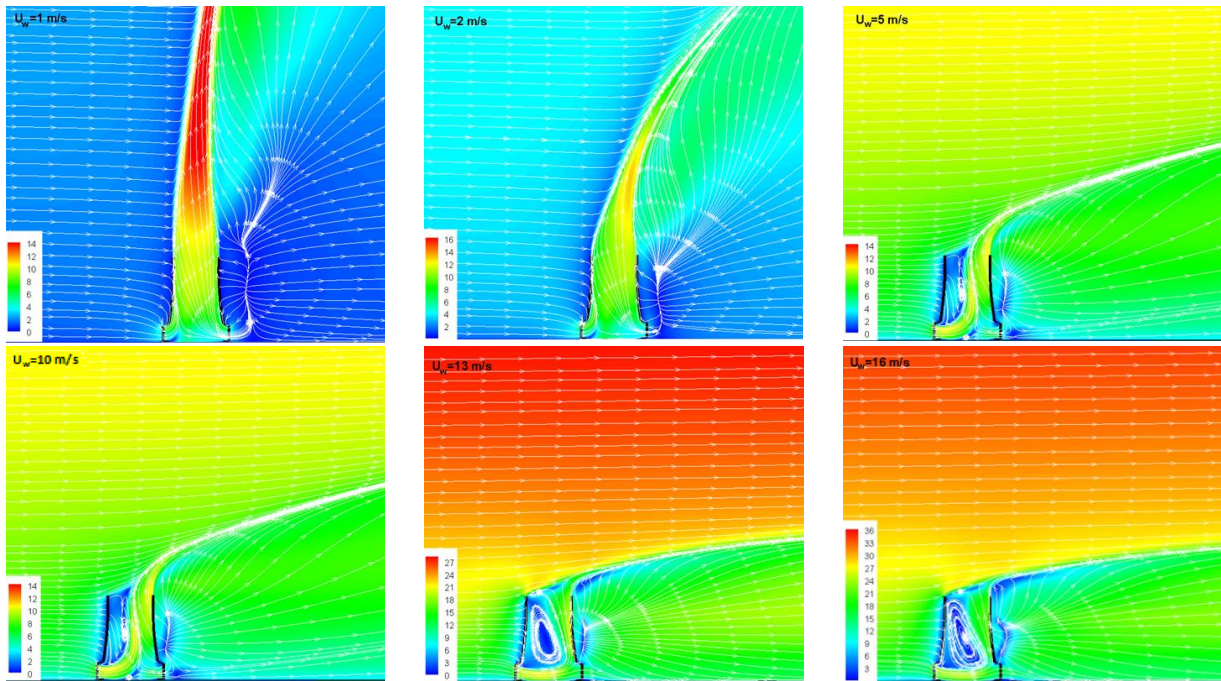
شکل ۱۶ خطوط مسیر و توزیع مقدار سرعت (m/s) در صفحه عمودی میانی برج
