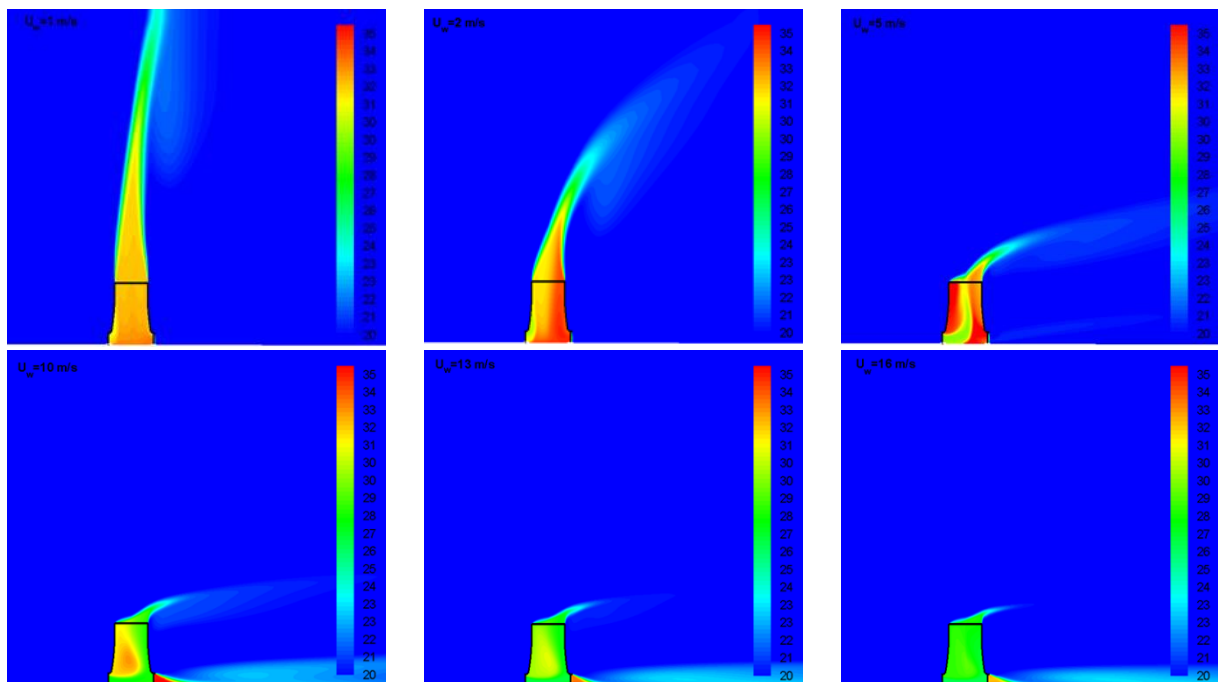
شکل ۱۵) توزیع دما (°C) در صفحه عمودی میانی برج
