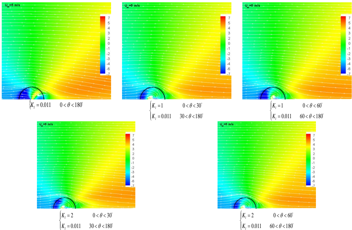
شکل ۲۴) توزیع مؤلفه شعاعی سرعت (m/s) و خطوط مسیر در صفحه افقی به ارتفاع ۱۲m (عبوری از میان ارتفاع رادیاتورها) در سرعت باد ۵m/s با لوره‌های نیمه‌باز
