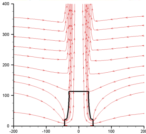
شکل ۸) خطوط جریان و بردارهای سرعت هوا برای ITD=۲۹
