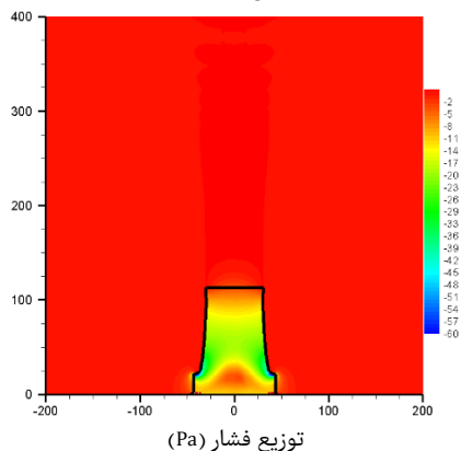
شکل ۷) توزیع فشار نسبی، دما و سرعت عمودی هوا در داخل و بیرون برج برای ITD=۲۹
