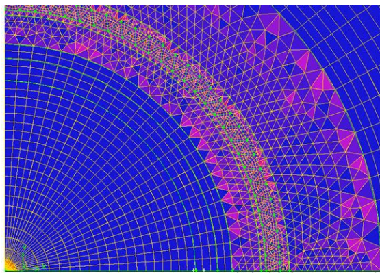
شکل ۲) شبکه ایجاد شده برای برج خنک‌کن و محیط اطراف آن
