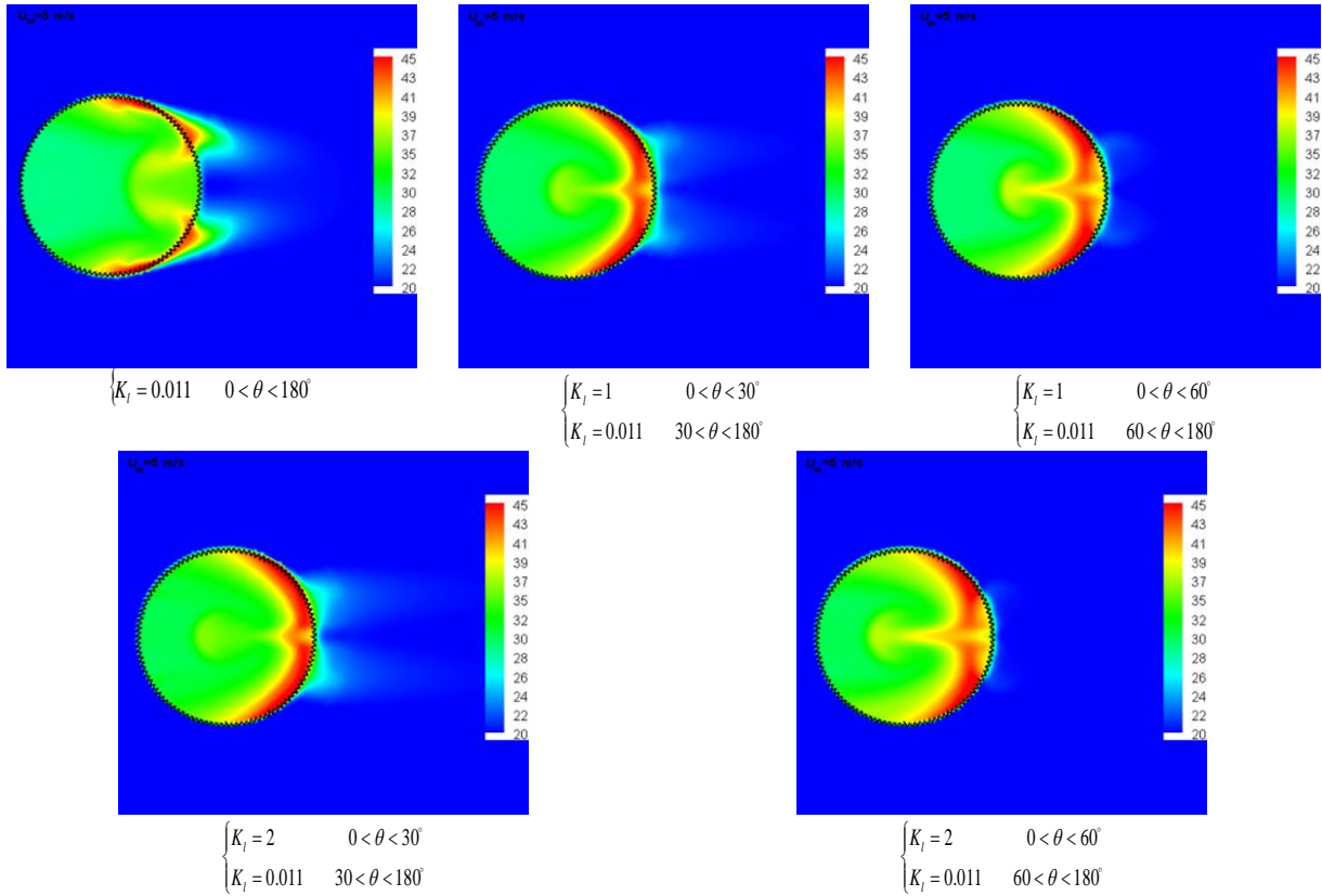
شکل ۲۳) توزیع دما (°C) در صفحه افقی به ارتفاع ۱۲m (عبوری از میان ارتفاع رادیاتورها) در سرعت باد ۵m/s با لوره‌های نیمه‌باز
