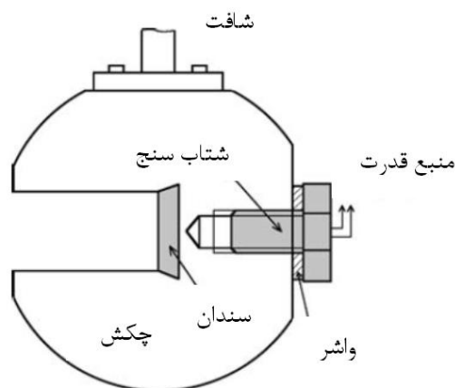
شکل ۱) طرح شماتیک نصب شتاب‌سنج روی چکش در آزمایش شارپی [۸]
