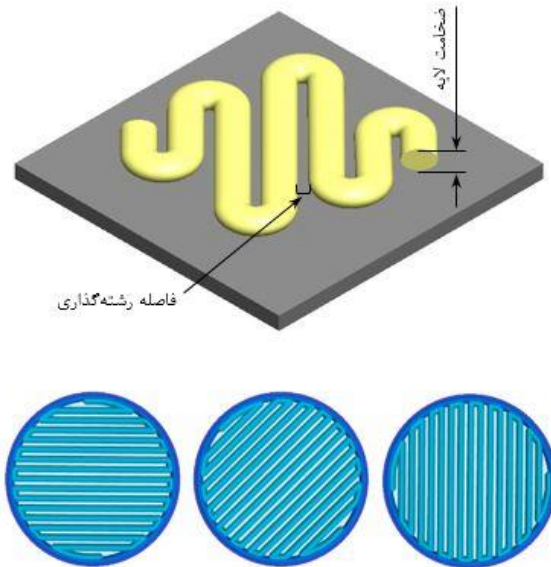
شکل ۱) متغیرهای فرآیند (شکل بالا): متغیرهای فاصله رشته‌گذاری و ضخامت لایه، شکل پایین: متغیر زاویه رشته‌گذاری در وضعیت‌های متفاوت)
