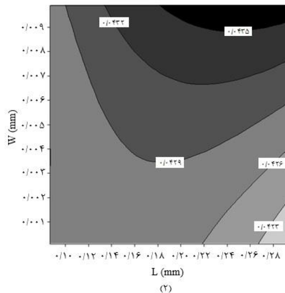
شکل 9) نمودار اثر متقابل متغیرهای ضخامت لایه و فاصله رشته‌گذاری بر نرخ سایش
