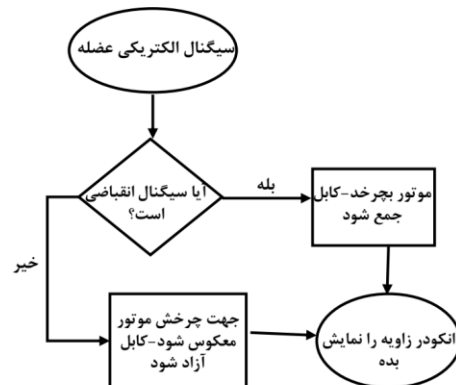
شکل ۵) فلوچارت کنترل با کمک سیگنال زیستی
