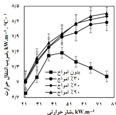
شکل ۷) مقایسه‌ی تغییرات فراصوت بر ضریب انتقال حرارت در محلول نمکی ۴۰ g.l -1
