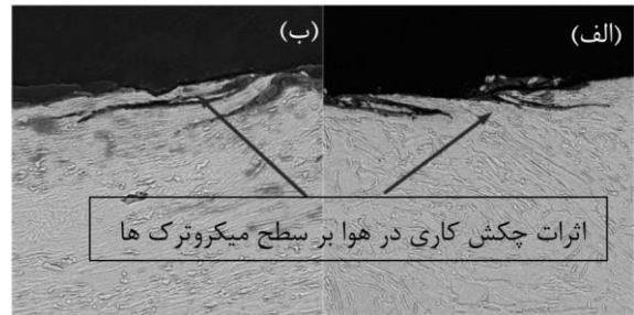
شکل ۹) (الف) - ترک در نمونه چکش کاری نشده (ب) - تأثیر چکش کاری فراصوتی در هوا بر روی ترک سطحی
