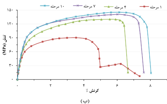
شکل ۱۰) منحنی تنش-کرنش کامپوزیت GLARE ساخته شده از الف) آلومینیوم آنیل شده و ب) آلومینیوم ARB ساخته شده با مراحل مختلف
