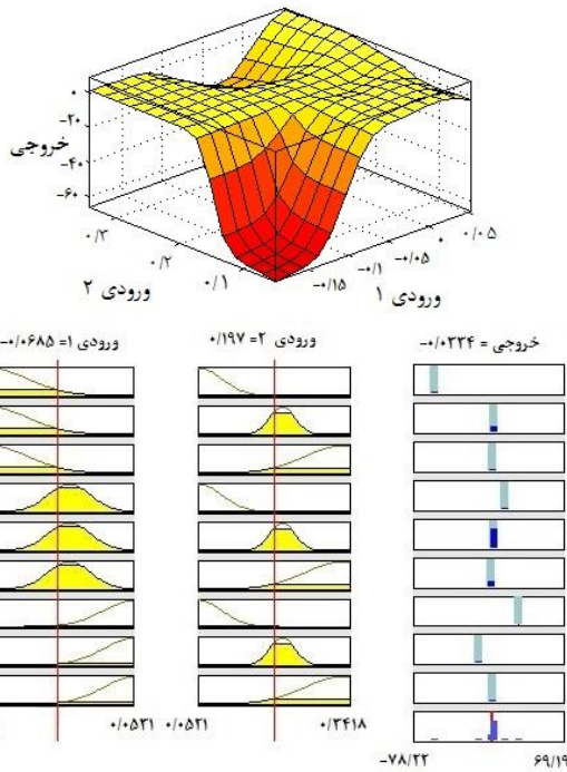
شکل ۹) نمودار قوانین فازی سطوح در فرآیند مدل سازی ANFIS
