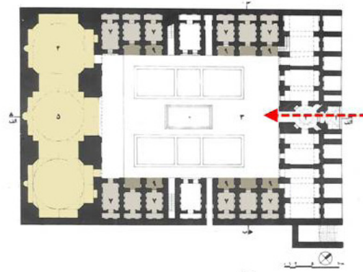
تصویر شماره ۹: برش افقی طبقه همکف؛ مأخذ: حاجی قاسمی، ۱۳۷۸: ۱۴۸
