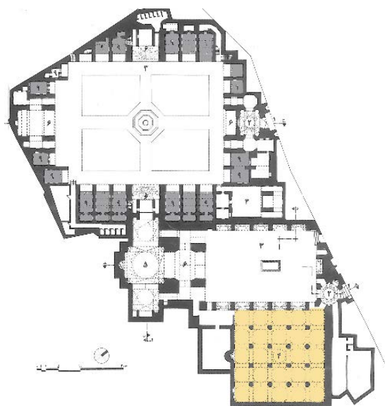
تصویر شماره ۱۳: برش افقی طبقه همکف، مأخذ: حاجی قاسمی، ۱۳۷۷: ۴۲.
