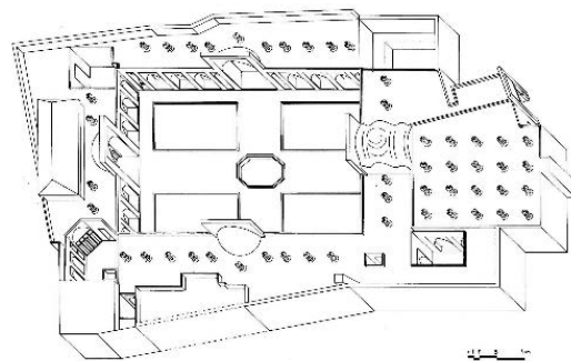
تصویر شماره ۵: تصویر سه بعدی گنجنامه مأخذ: بناهای مذهبی تهران، ۱۳۷۷: ۱۲۵.
