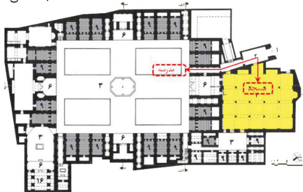
تصویر شماره ۴: برش افقی طبقه همکف، در پلان مشاهده می شود که در هشتی ورودی فضای مسجد و مدرسه از هم تفکیک شده است. مأخذ: گنجنامه بناهای مذهبی تهران، ۱۳۷۷: ۱۲۷.
