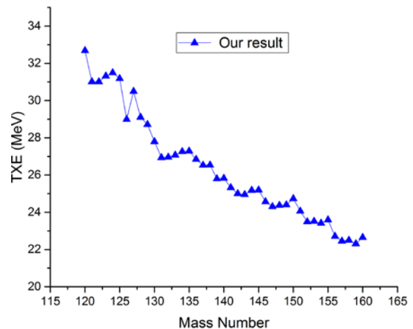
شکل ۱۰. انرژی تحریکی کل محاسبه شده برای شکافت نوترونی اورانیم-۲۳۹.
