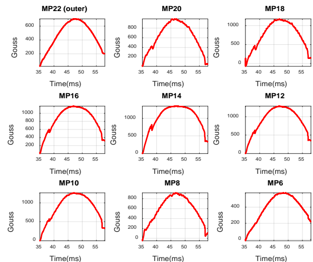
شکل ۱۱. نمایش سیگنال‌های پروب‌های مغناطیسی دیواره خارجی بعد از اعمال پیش‌پردازش برای شات ۲۸.
