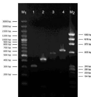
شکل ۲- الکتروفورز محصولات حاصل از تکثیر گروه‌های اختصاصی agr بر روی ژل آگاروز. چاهک M 1 : مارکر GeneRuler™ 100 bp DNA ladder؛ چاهک ۱: agr I (441 bp)؛ چاهک ۲: agr II (575 bp)؛ چاهک ۳: agr III (323 bp)؛ چاهک ۴: agr IV (659 bp)؛ چاهک ۵: چاهک plus marker؛ چاهک M 2 : مارکر \Phi X174DNA/ BsuRI ( HaeIII ) marker.
