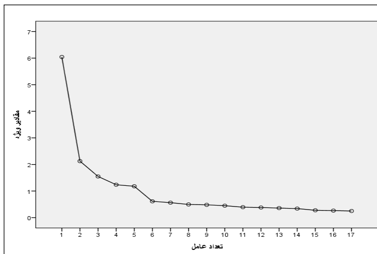
شکل ۲- نمودار سنگریزه‌ای برای تعیین تعداد عامل‌ها 2019, Research findings, Source:
