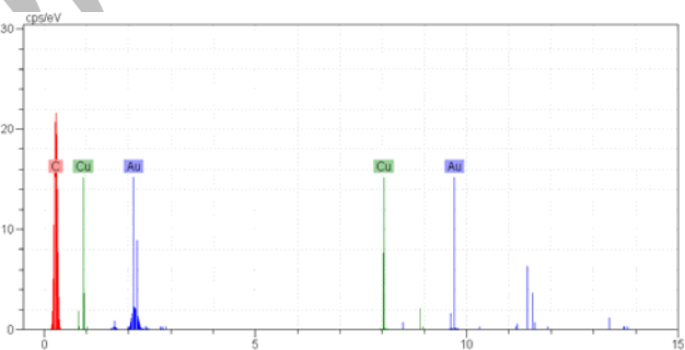
شکل ۴- مقدار عناصر شمارش شده در نمونه‌ی پلی اتیلنی که در واحد زمان به آشکارساز می‌رسد.
