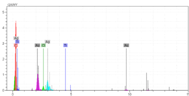
شکل ۶- مقدار عناصر شمارش شده در نمونه‌ی پلی اتیلن همپوشانی شده با نانو ذرات نقره و دی اکسید تیتانیوم که در واحد زمان به آشکارساز می‌رسد.
