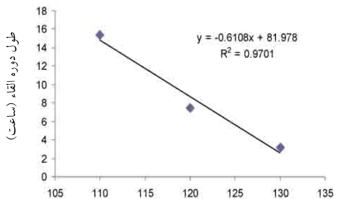
شکل ۹ - تغییرات طول دوره‌ی القاء بر حسب افزایش دما در روغن پسته
