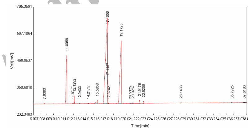
شکل ۵ - کروماتوگرام GC ترکیب اسیدهای چرب روغن پسته
