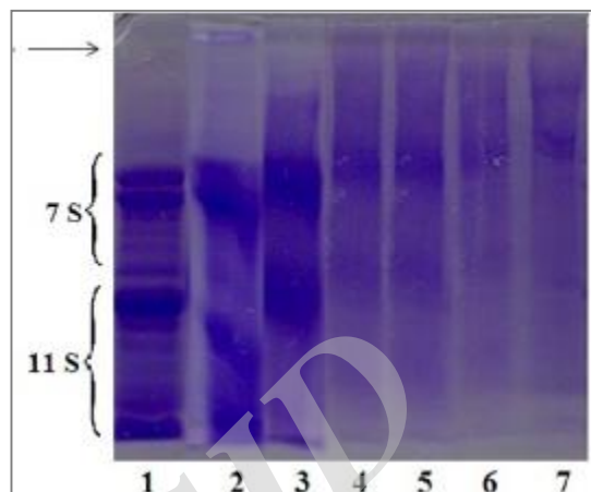
شکل 1- الگوی الکتروفورز پروتئین های سویای کانژوگه شده با دکستران در دمای 60^{\circ}\text{C} ، \text{pH} : 8/5 و زمان های مختلف بر روی ژل اکریل آمید
