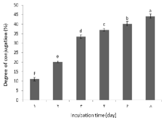
شکل 2- درصد جایگزینی گروه های آمینی در کانژوگه های تیمار شده در دمای 60^{\circ}\text{C} ، \text{pH} : 8/5 و زمان های مختلف (هر ستون نمایانگر میانگین \pm انحراف معیار برای سه تکرار می باشد)
