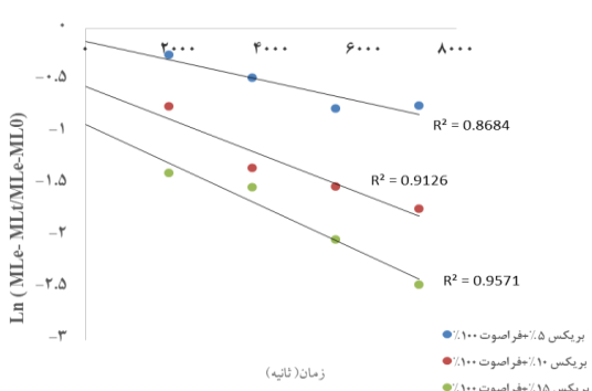
شکل ۷- نمودار تغییرات لگاریتمی مقادیر از دست دادن آب (ML) در برابر زمان t در غلظت های ۱۰، ۵ و ۱۵ درصد و فراصوت ۵۰ (الف) و ۱۰۰ (ب)
