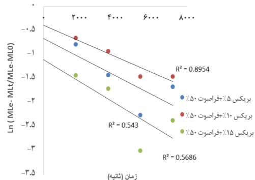
شکل ۷- نمودار تغییرات لگاریتمی مقادیر از دست دادن آب (ML) در برابر زمان t در غلظت های ۱۰، ۵ و ۱۵ درصد و فراصوت ۵۰ (الف) و ۱۰۰ (ب)
