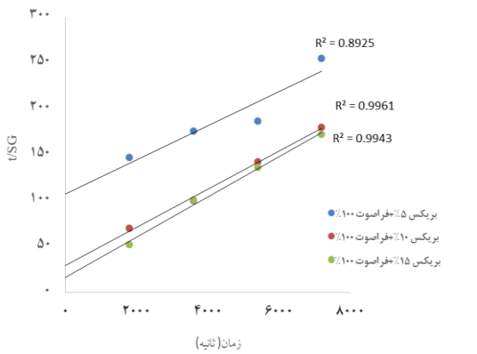
شکل ۶- نمودار خطی مدل آزارا برای تعیین مقادیر SG e در غلظت های ۱۰، ۵ و ۱۵ درصد و فراصوت ۵۰ (الف) و ۱۰۰ (ب)
