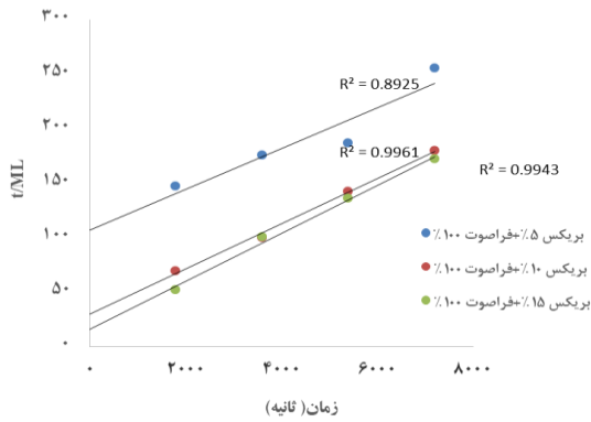
شکل ۵- نمودار خطی مدل آزارا برای تعیین مقادیر MLe در غلظت های ۱۰، ۵ و ۱۵ درصد و فراصوت ۵۰ (الف) و ۱۰۰ (ب)
