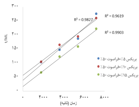
شکل ۵- نمودار خطی مدل آزارا برای تعیین مقادیر MLe در غلظت های ۱۰، ۵ و ۱۵ درصد و فراصوت ۵۰ (الف) و ۱۰۰ (ب)
