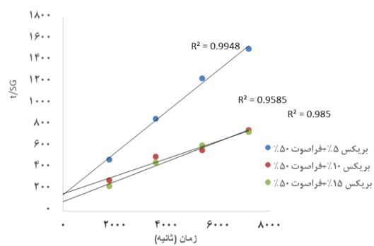
شکل ۶- نمودار خطی مدل آزارا برای تعیین مقادیر SG e در غلظت های ۱۰، ۵ و ۱۵ درصد و فراصوت ۵۰ (الف) و ۱۰۰ (ب)
