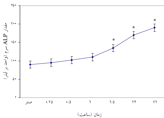
نمودار شماره ۲- نمودار تغییرات ALP سرم بعد از بیهوشی با پروپوفول در زمانهای مختلف. *: p < 0/05 در مقایسه با زمان صفر می باشد.
