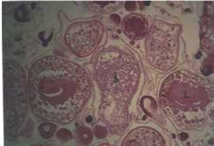
شکل شماره ۲- تصویر میکروسکوپی از تخمدان ماهی کپور معمولی (در مجاورت با سولفات مس) (درشتنمایی X=40) ۱- Primary Oocyte (Po) ۲- Secondary Oocyte (So) ۳- دزیره شدن تخمک‌ها (Oocyte Degeneration)
