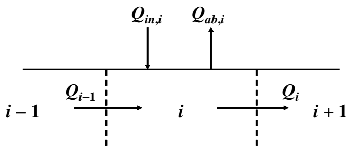
شکل ۲: معادله جابجایی- انتشار یک بعدی.
