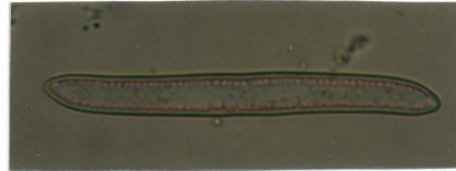
Nitzschia
