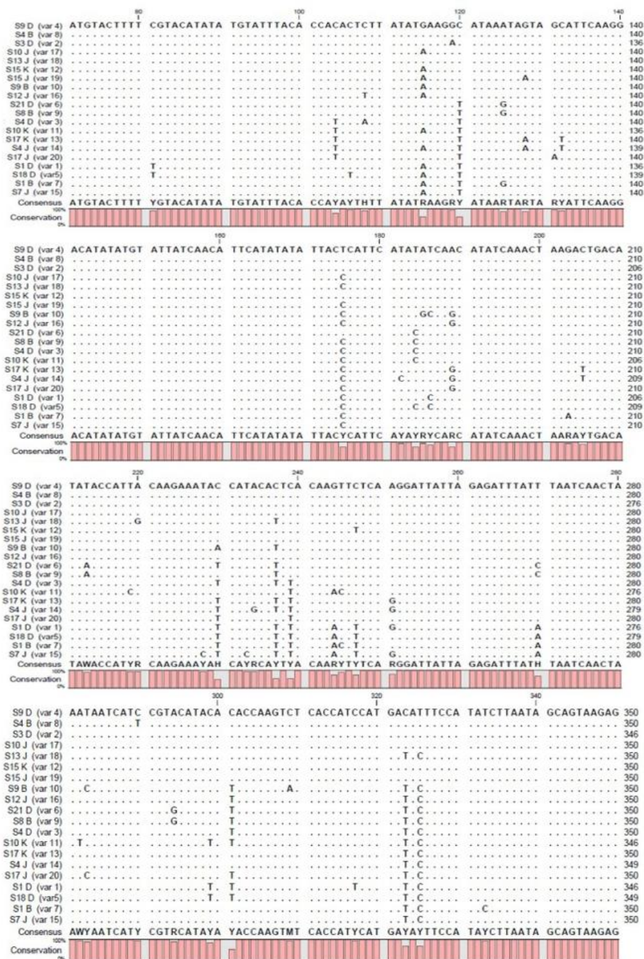
شکل ۴: هم ترازوی ۲۰ نمونه منتخب که توسط نرم افزار CLC Viewer انجام و محدوده تفاوتها آورده شده است.
