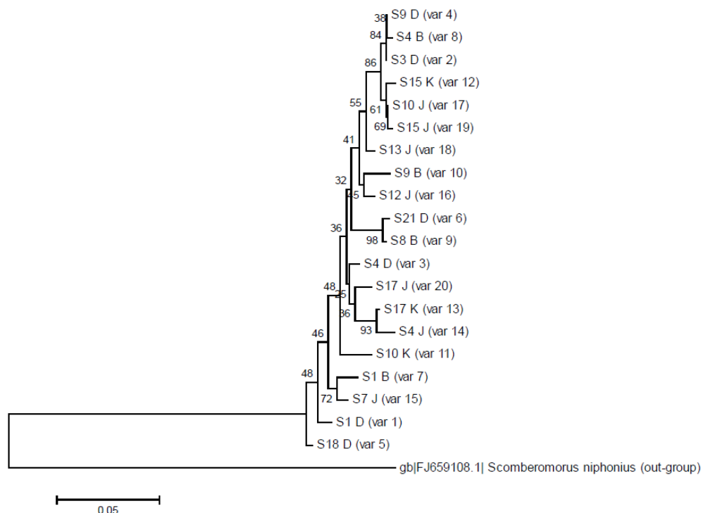
شکل ۵: درخت فیلوژنی ۲۰ نمونه منتخب، شماره دسترسی به توالی های ثبت شده در بانک ژنی NCBI برای نمونه‌های S4B، S1D، S4J، S15K به ترتیب (LC101261.1 - LC101262.1 - LC101263.1 - LC101264.1، S17K، (LC101268.1) S3D، (LC101270.1) می‌باشند و باقی در حال ثبت شدن هستند.
