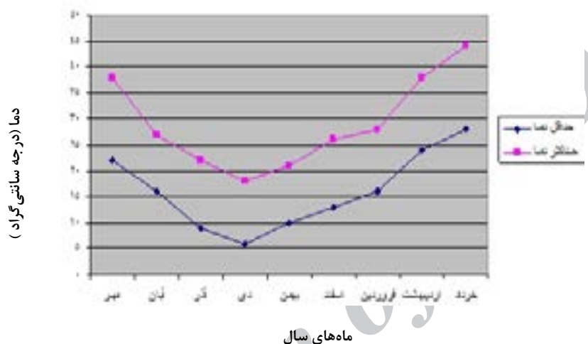
شکل ۱: روند دمای میانگین در مدت زمان انجام تحقیق در ایستگاه اهواز
