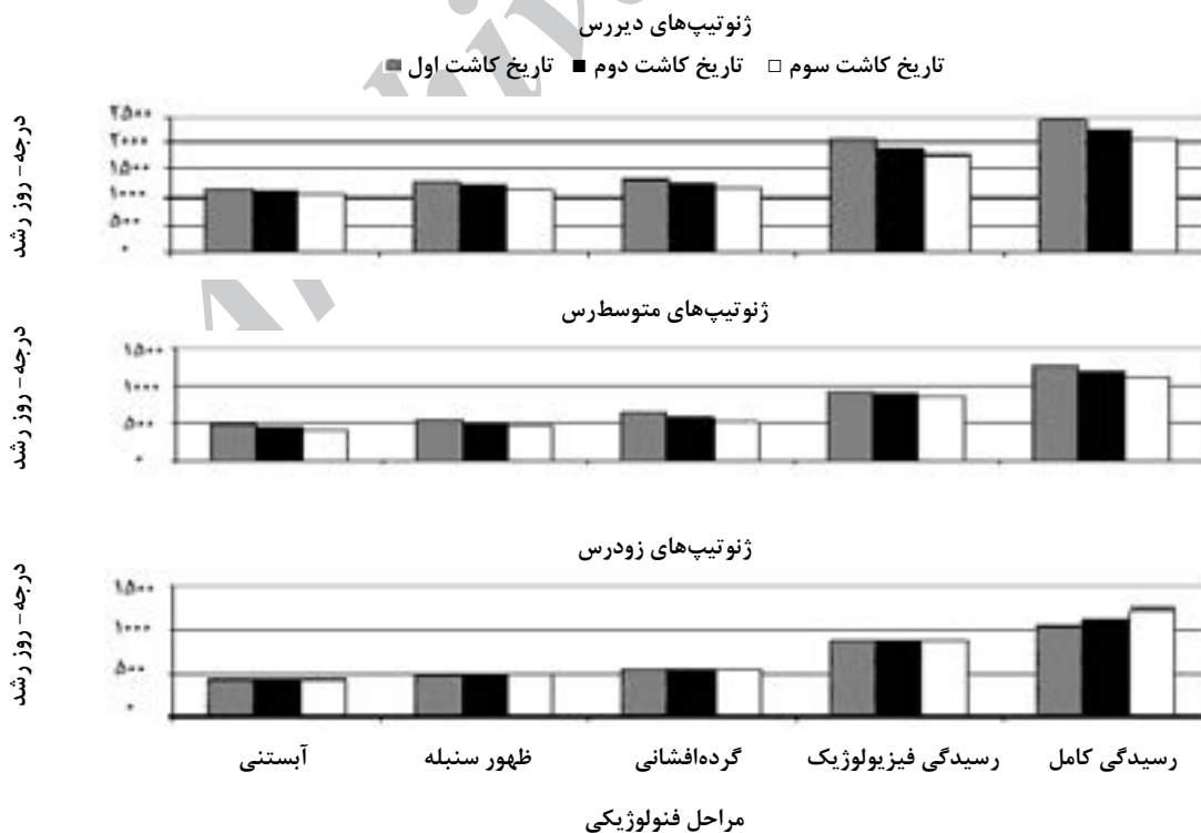
شکل ۲: روند تغییرات درجه-روز رشد تجمعی از کاشت تا مراحل مختلف فنولوژیکی در ژنوتیپ‌های مختلف. اولین تاریخ کاشت ۸/۵، ۸/۲۵ و ۹/۲۵ و به ترتیب به فاصله ۱۰، ۱۵ و ۱۰ روز پس از اولین تاریخ کاشت در آزمایش اول، دوم و سوم می‌باشد.
