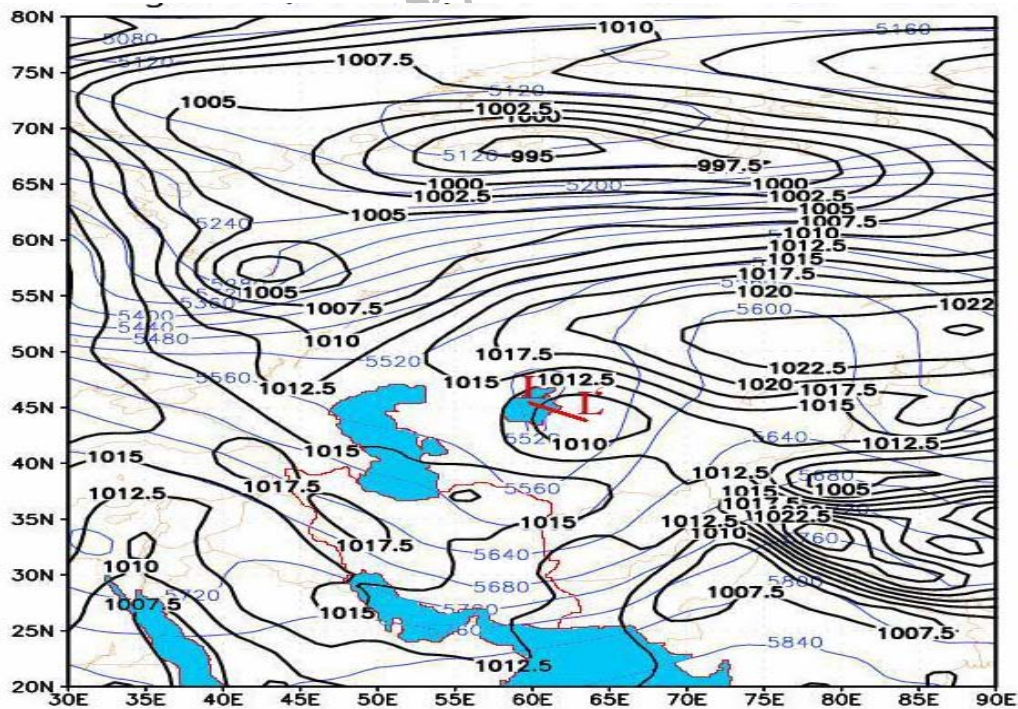
شکل ۱۱- خطوط مشکی، خطوط هم فشار در سطح متوسط دریا و خطوط آبی، خطوط هم ارتفاع 500\text{ hpa} می باشند. خط قرمز مرکز چرخند مورد نظر ( L' ) را به مرکز کم ارتفاع 500\text{ hpa} وصل می کند. (چرخند L در اینجا کاملاً از بین رفته و تنها L' باقی مانده است). (ساعت (UTC) ۰۰ روز ۲ آوریل ۲۰۰۹).
