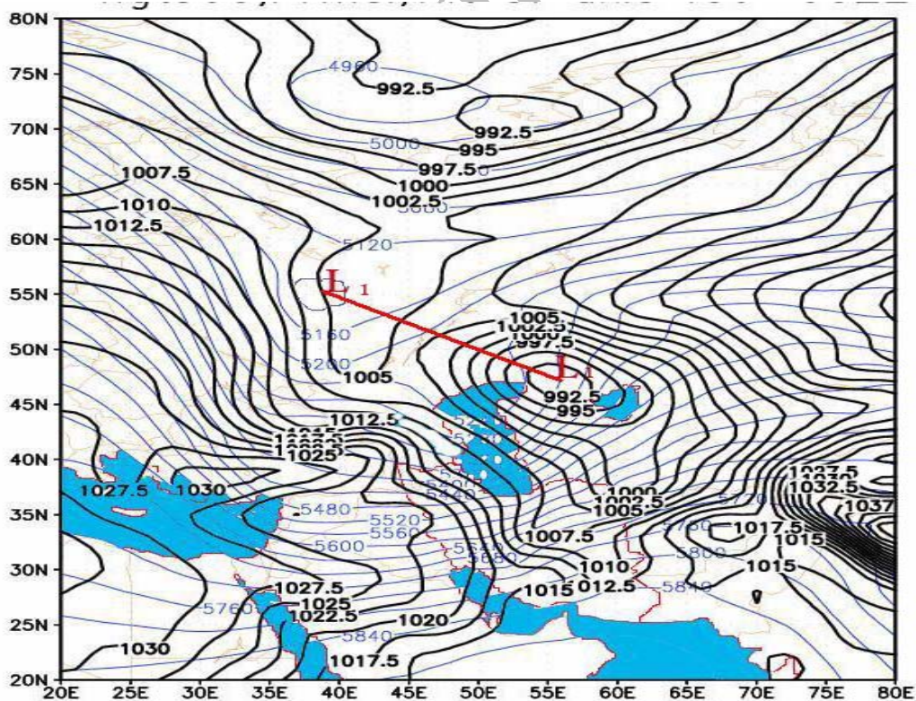
شکل ۷- خطوط مشکی، خطوط هم فشار در سطح متوسط دریا و خطوط آبی، خطوط هم ارتفاع hpa ۵۰۰ می باشند. خط قرمز مرکز چرخند مورد نظر (L 1 ) را به مرکز کم ارتفاع hpa ۵۰۰ وصل می کند. (ساعت UTC) روز ۲۰ فوریه ۲۰۰۸.
