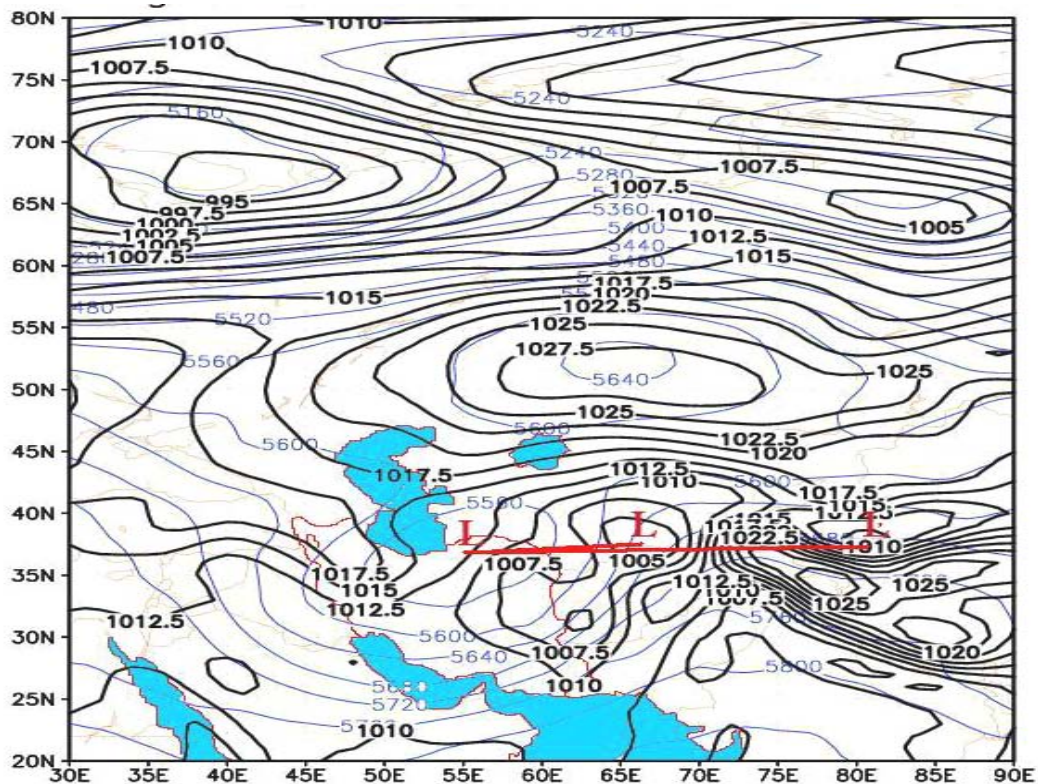
شکل ۱۰- خطوط مشکی، خطوط هم فشار در سطح متوسط دریا و خطوط آبی، خطوط هم ارتفاع 500\text{ hpa} می باشند. خطوط قرمز مرکز چرخند های مورد نظر ( L, L' ) (چرخند بررسی شده در جدول سوم است). را به مرکز کم ارتفاع 500\text{ hpa} وصل می کند. (ساعت (UTC) ۰۰ روز ۱ آوریل ۲۰۰۹)
