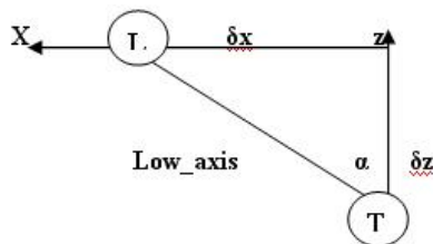
شکل ۴- خم شدن محور فضایی در یک نظام چرخندی
