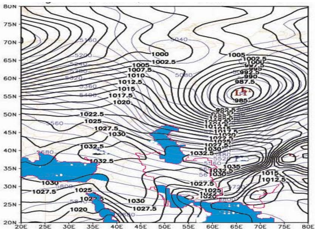
شکل ۸- خطوط مشکی، خطوط هم فشار در سطح متوسط دریا و خطوط آبی، خطوط هم ارتفاع 500\text{ hPa} می باشند. خط قرمز مرکز چرخند مورد نظر ( L_1 ) را به مرکز کم ارتفاع 500\text{ hPa} وصل می کند. (ساعت (UTC) ۱۸ روز ۲۱ فوریه ۲۰۰۸).
