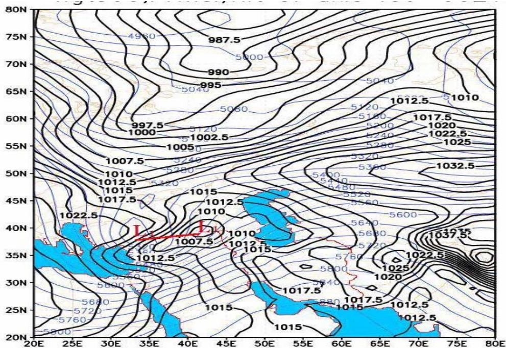
شکل ۶- خطوط مشکی، خطوط هم فشار در سطح متوسط دریا و خطوط آبی، خطوط هم ارتفاع hpa ۵۰۰ می باشند. خط قرمز مرکز چرخند مورد نظر (L 1 ) را به مرکز کم ارتفاع hpa ۵۰۰ وصل می کند. (ساعت UTC) روز ۱۹ فوریه ۲۰۰۸.
