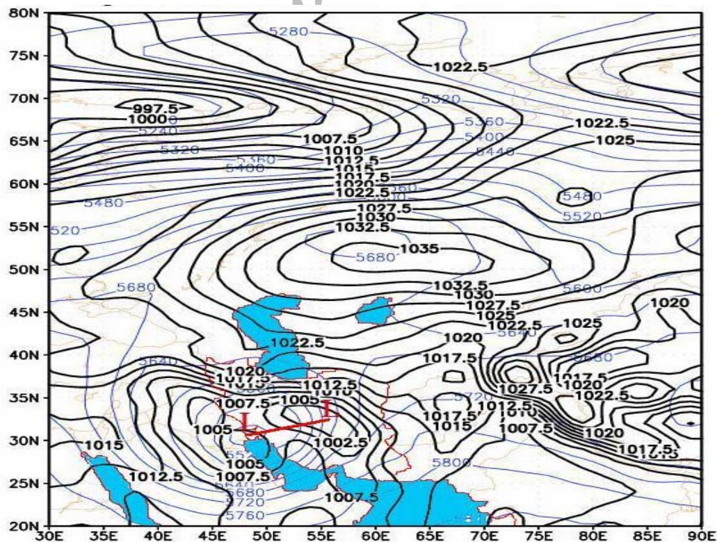
شکل ۹- خطوط مشکی، خطوط هم فشار در سطح متوسط دریا و خطوط آبی، خطوط هم ارتفاع 500\text{ hPa} می باشند. خط قرمز مرکز چرخند مورد نظر ( L ) را به مرکز کم ارتفاع 500\text{ hPa} وصل می کند. (ساعت (UTC) ۰۰ روز ۳۱ مارس ۲۰۰۹)
