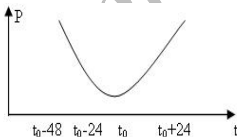
شکل ۳- برون یابی نموداری از تکامل تدریجی یک چرخند.
