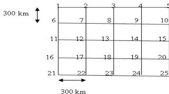
شکل ۲- شبکه بندی برای محاسبه‌ی کارمایه‌ی نهفته‌ی در دست رس مرکز عمیق شدن در نقطه ۱۳ می باشد.
