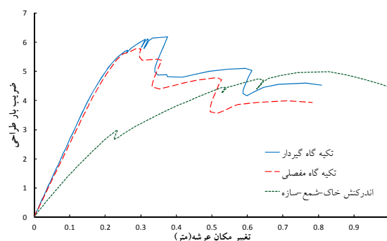
شکل ۱۱- نمودار نیرو-تغییر مکان سکو LQX در راستای قطری
