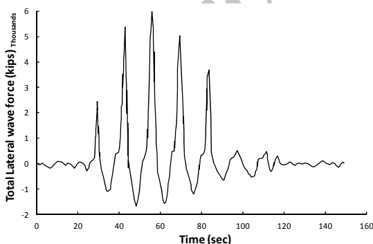
شکل ۱- تاریخچه زمانی نیروهای ثبت شده برای یک نمونه سکوی طوفان الیا [۱۷]
