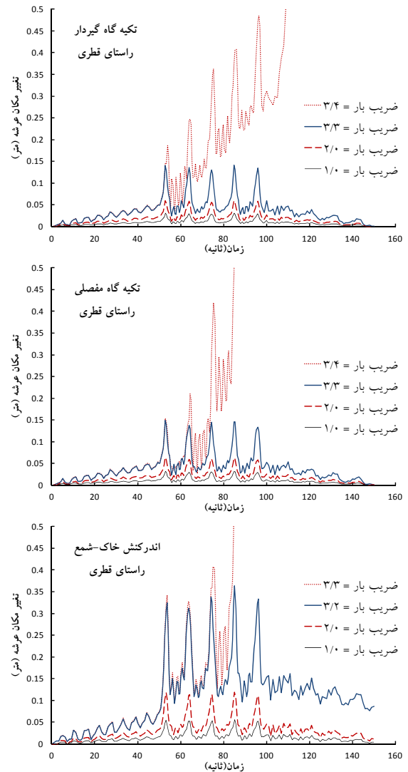
شکل ۱۴- تغییر مکان عرشه سکوی LQ تحت بارگذاری در راستای قطری
