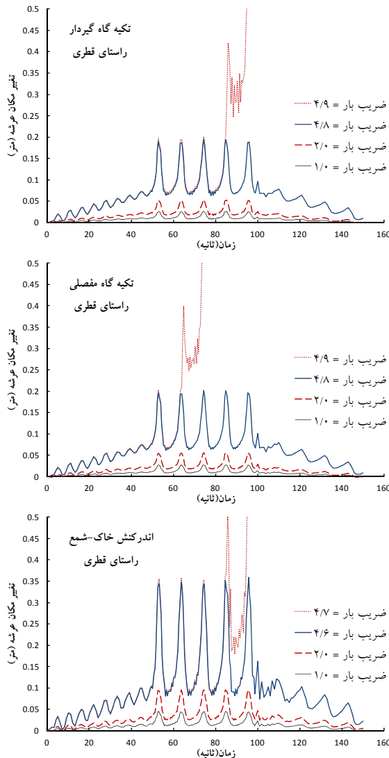
شکل ۱۵- تغییر مکان عرشه سکوی LQX تحت بارگذاری در راستای قطری
