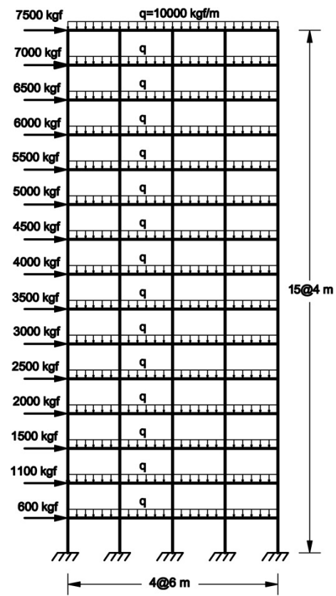
شکل ۱۱- قاب ساختمانی ۱۵ طبقه
