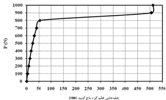
شکل ۱۶- مسیر ایستایی خرپای گنبدی
