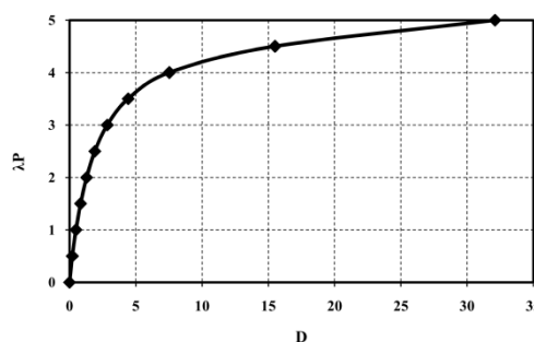
شکل ۸- مسیر ایستایی خرابای چن
