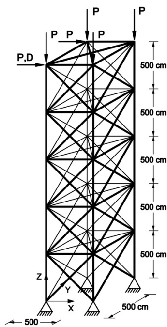
شکل ۱۹- پایه خرپایی
