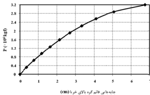
شکل ۲- مسیر ایستایی خرابی دو عضوی
