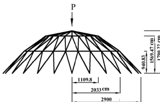
شکل ۱۵- خرپای گنبدی
