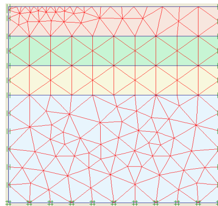
شکل ۶- نمونه‌ای از شبکه‌بندی محدوده
