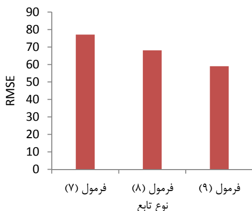
شکل ۲۰- جذر خطای میانگین مربعات در توابع مختلف
