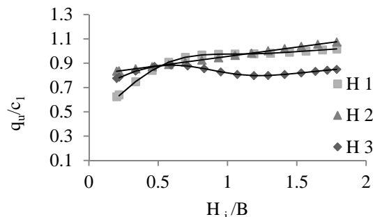
شکل ۱۵- اثر افزایش ضخامت لایه‌ها بر مقدار ظرفیت باربری
